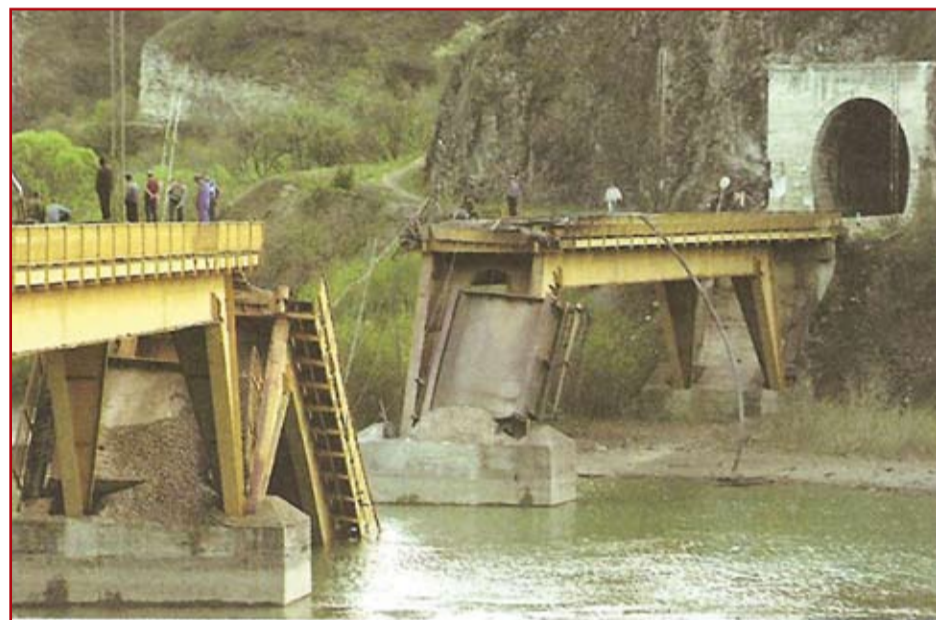
Железнички мост на реци Бистрици
